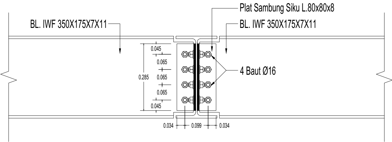
Pot - A. ( S 04 ) Skala 1:10
