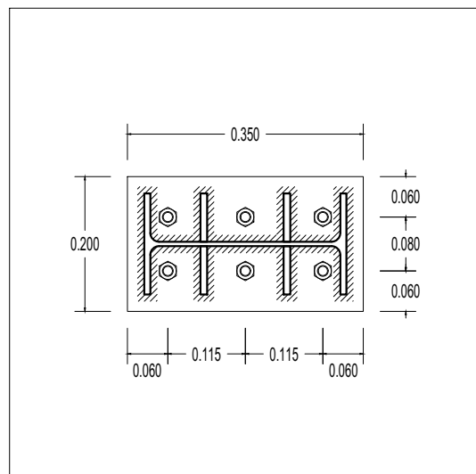
Det. - Sambungan ( 09 ) Skala 1:10
